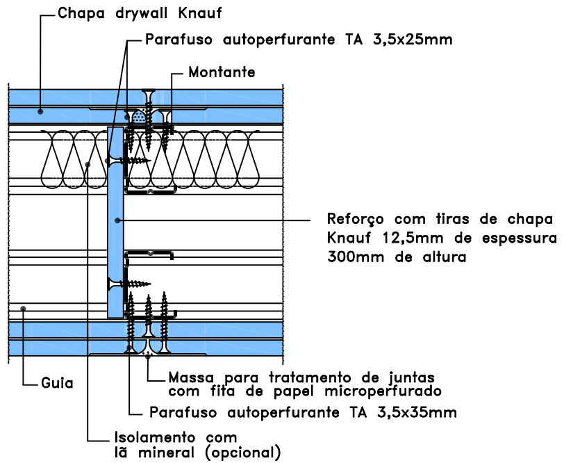
1 DETALHE - JUNTA DE CHAPAS ESTRUTURA SIMPLES - W116 SEM ESCALA
