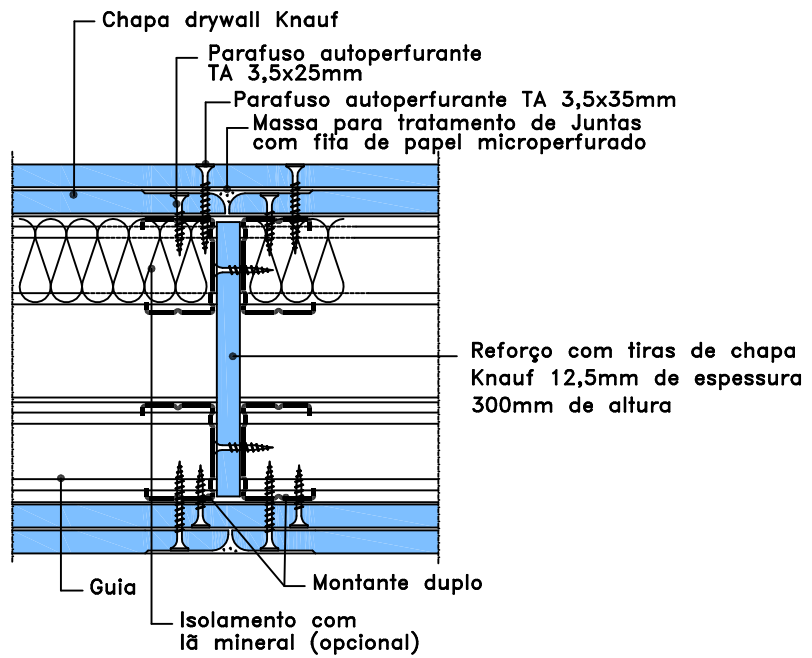
2 DETALHE - JUNTA DE CHAPAS ESTRUTURA DUPLA - W116 SEM ESCALA
