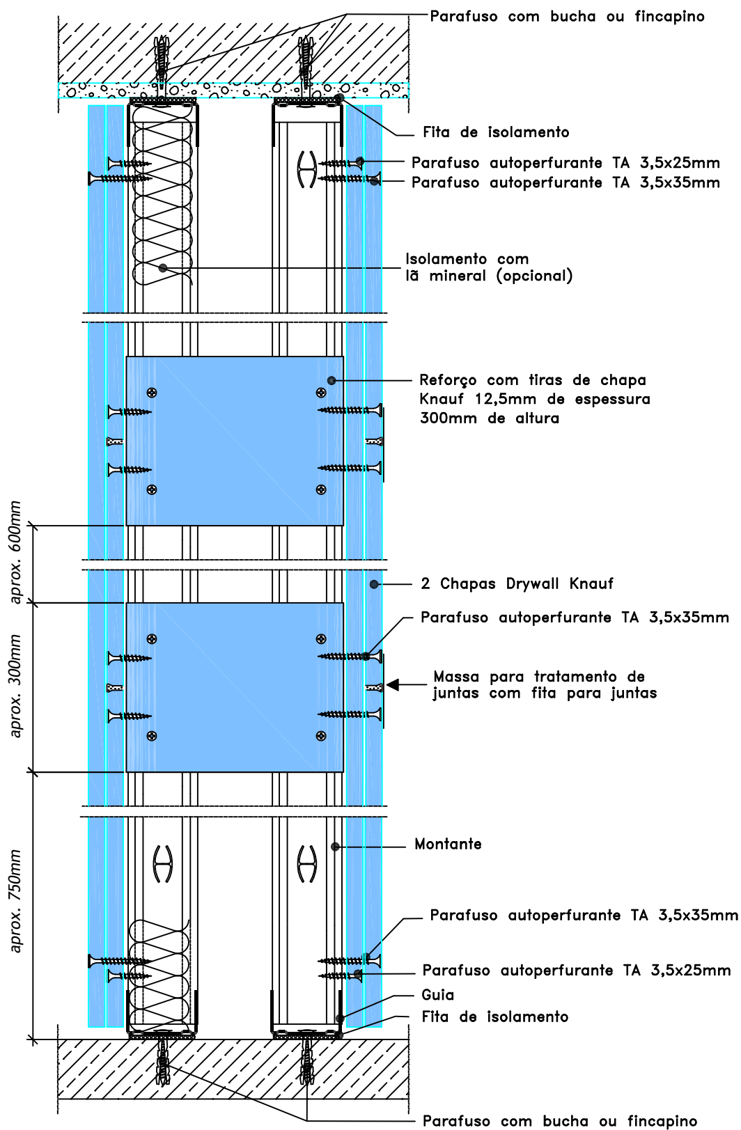
1 CORTE VERTICAL - W116 SEM ESCALA
